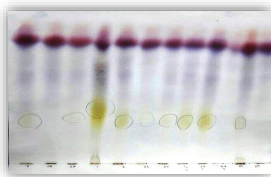
شکل ۱. پلیت TLC برای آنالیز نوع ایزومر دی آمینوپایمیلیک اسید در بین جدایه‌های اکتینوباکتر. لکه‌های بنفش (ارغوانی): اسید آمینه‌های موجود (به جز دی آمینوپایمیلیک اسید)، لکه‌های سبز زیتونی: مولکول‌های DAP. ایزومر R_f L کمتری نسبت به ایزومر meso داشته است.
