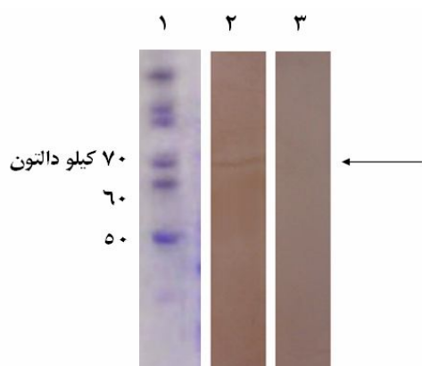
شکل 6. وسترن بلات پروتئین نو ترکیب فلاژین ویبریوکلرا؛ ستون 1: مارکر، ستون 2: وسترن بلات پروتئین نو ترکیب با سرم رت ایمن شده؛ ستون 3: کنترل منفی
