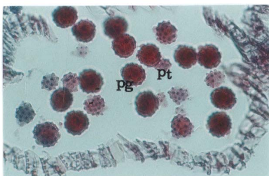
شکل ۲. برش عرضی بساک رسیده با دانه های گرده بالغ. با آراستار آگزینی خاردار. pg: دانه گرده و pt: لایه مغذی آمیبی، درشت نمایی ۴۰۰
